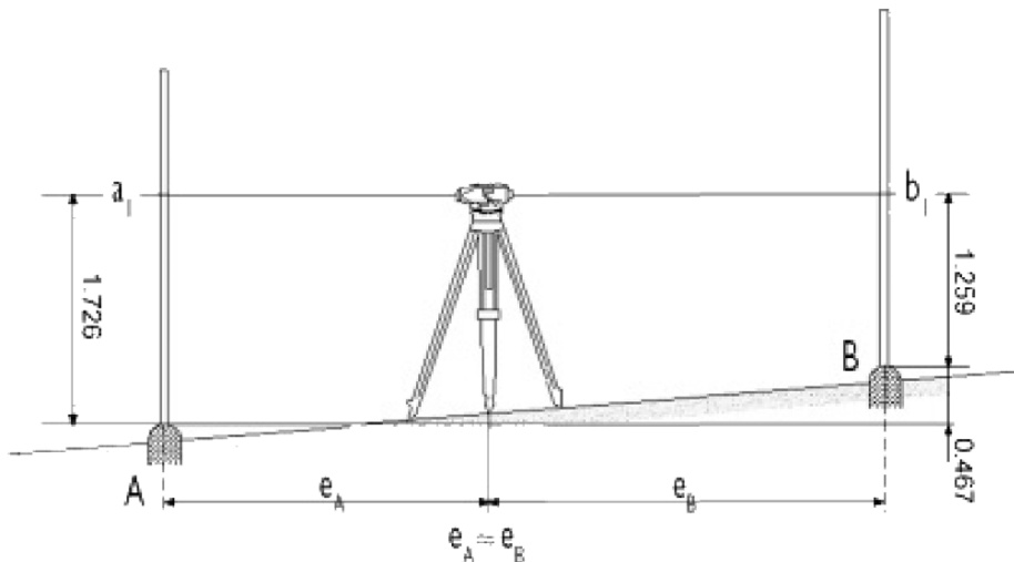
Рисунок 2: Нивелирование
